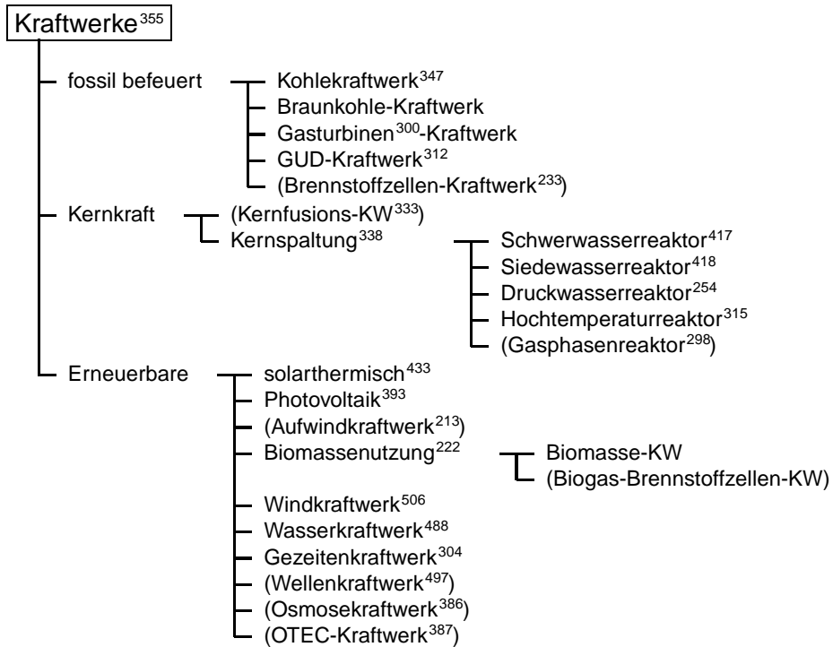
Abb. 2.10: Übersicht über die verschiedenen verfügbaren und experimentell untersuchten Kraftwerke Die in Klammern gesetzten Kraftwerkstypen sind nur „auf dem Reißbrett“ entworfen oder als Prototypen realisiert.
