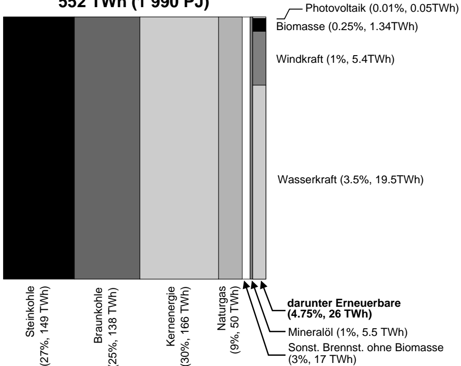
Abb. 2.9: Anteile der verschiedenen Energieträger an der jährlichen Stromerzeugung in Deutschland, 1998/1999
